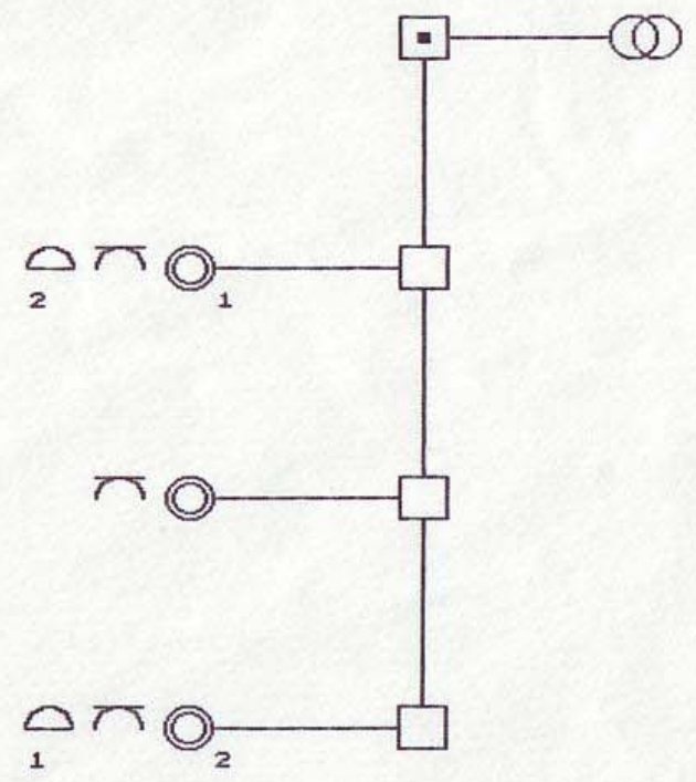
Schema unifilare
