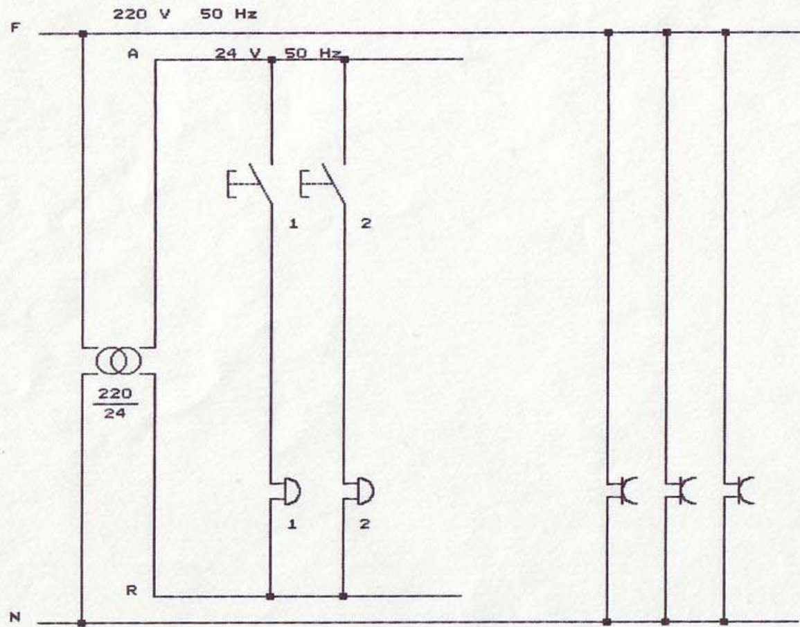
Schema funzionale
