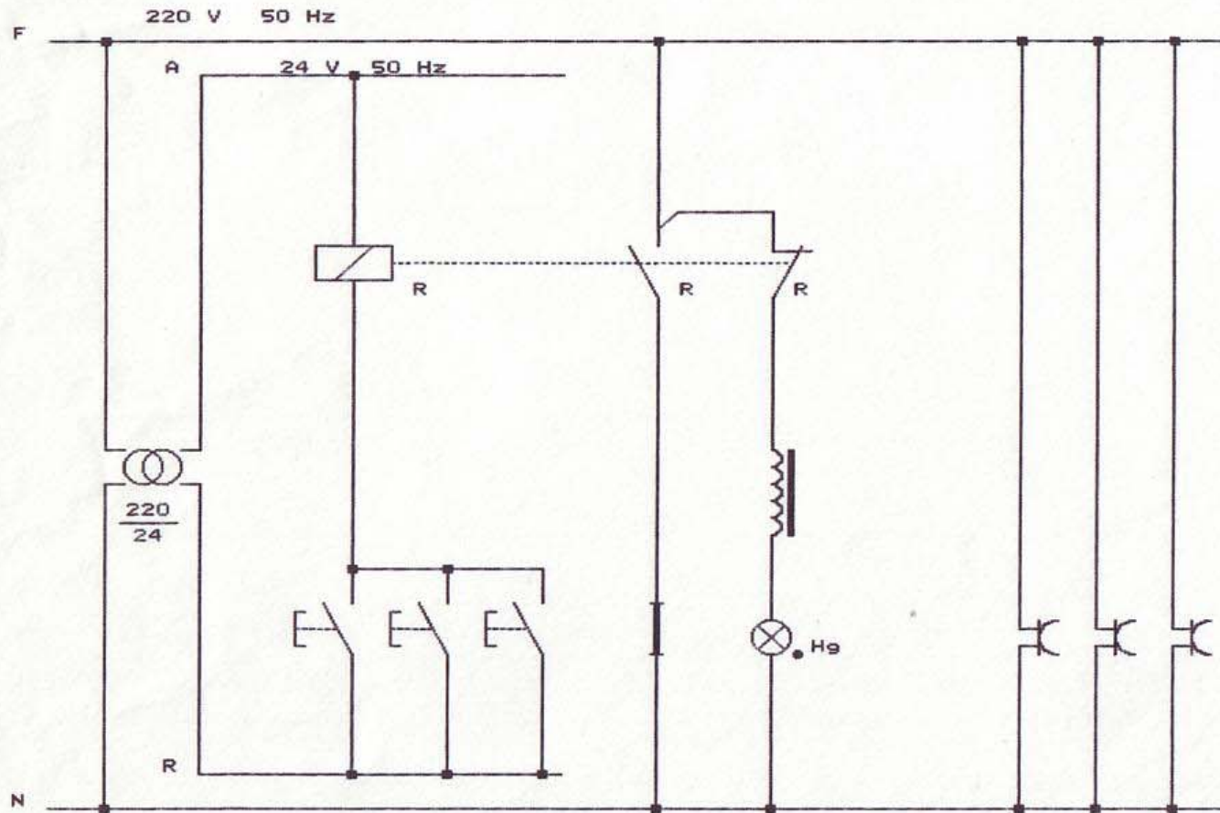
Schema funzionale
