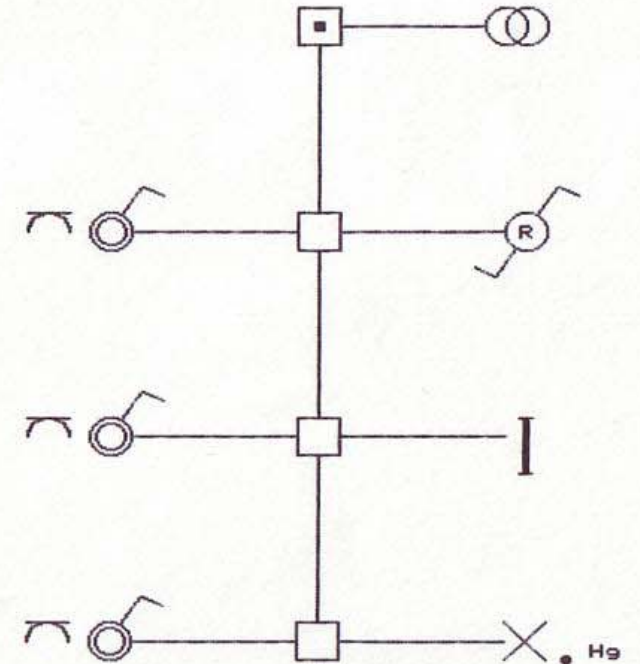
Schema unifilare
