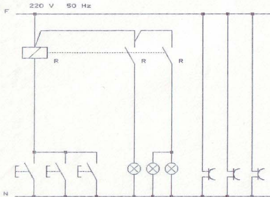
Schema funzionale
