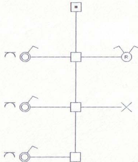
Schema unifilare
