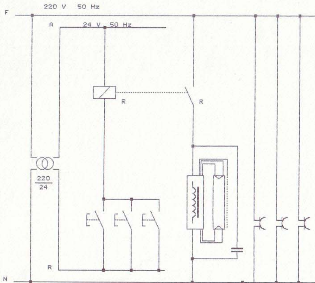
Schema funzionale
