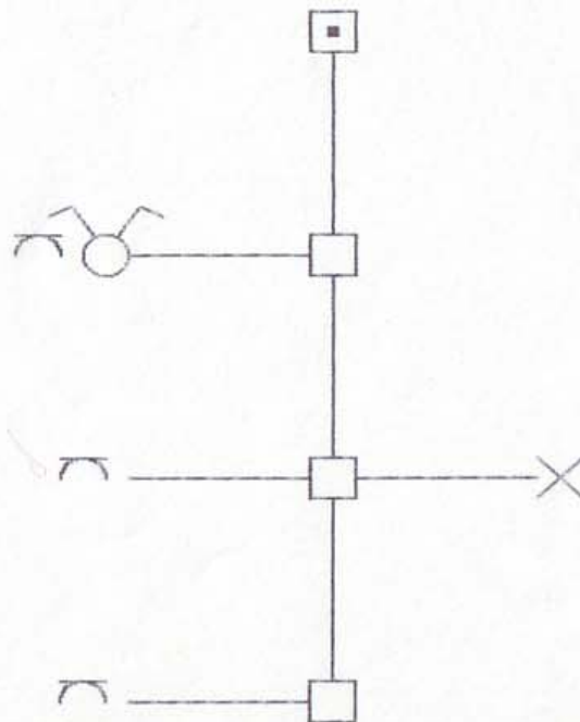
Schema unifilare
