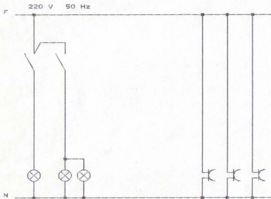
Schema funzionale
