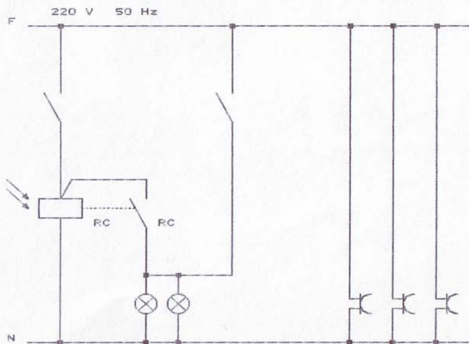
Schema funzionale
