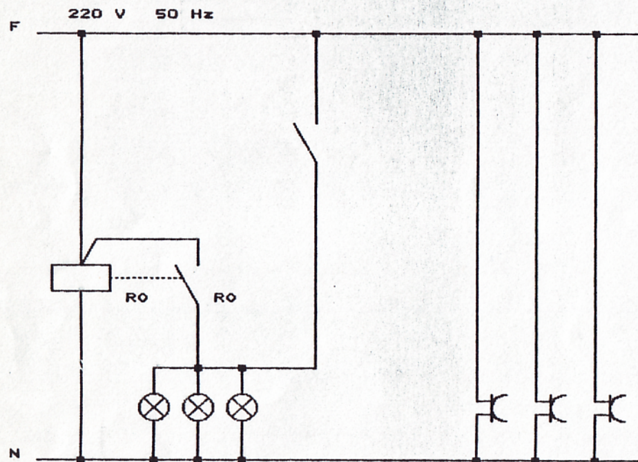
Schema funzionale
