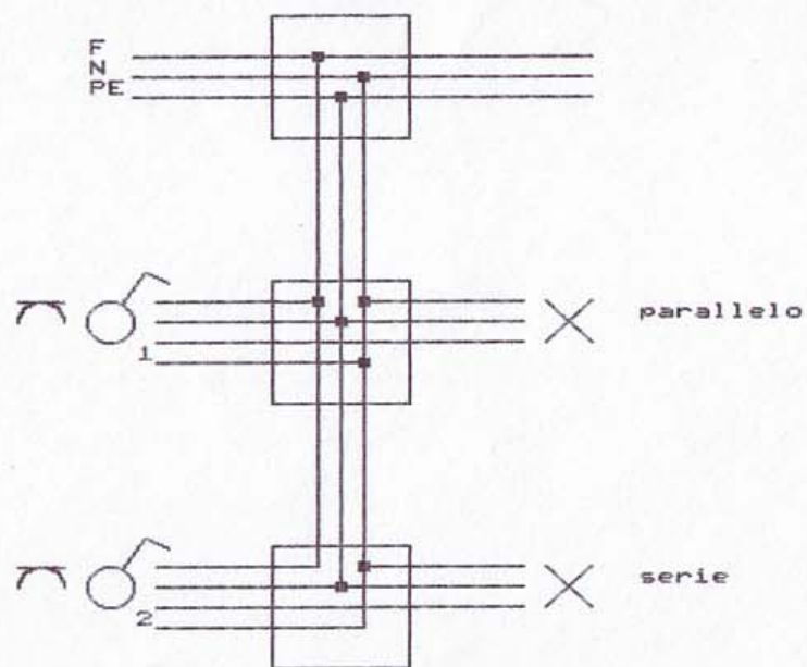
Schema multifilare
