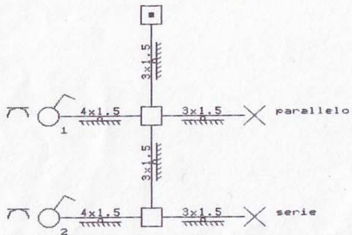
Schema unifilare
