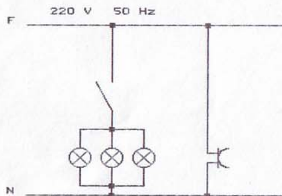
Schema funzionale
