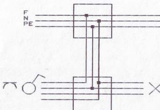
Schema multifilare
