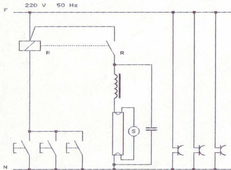
Schema funzionale
