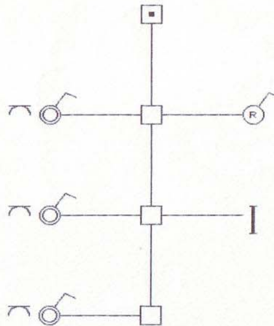
Schema unifilare
