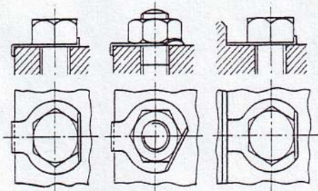
esempi di applicazione della rosetta di sicurezza con linguetta
