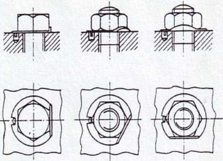
esempi di applicazione della rosetta elastica con nasello
