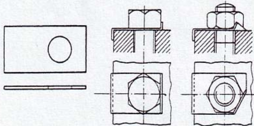
piastrina di sicurezza ed esempi di applicazione
