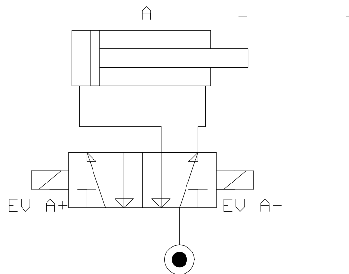
Schema di potenza
