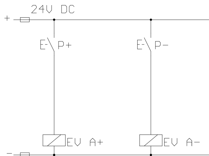
Schema di comando
