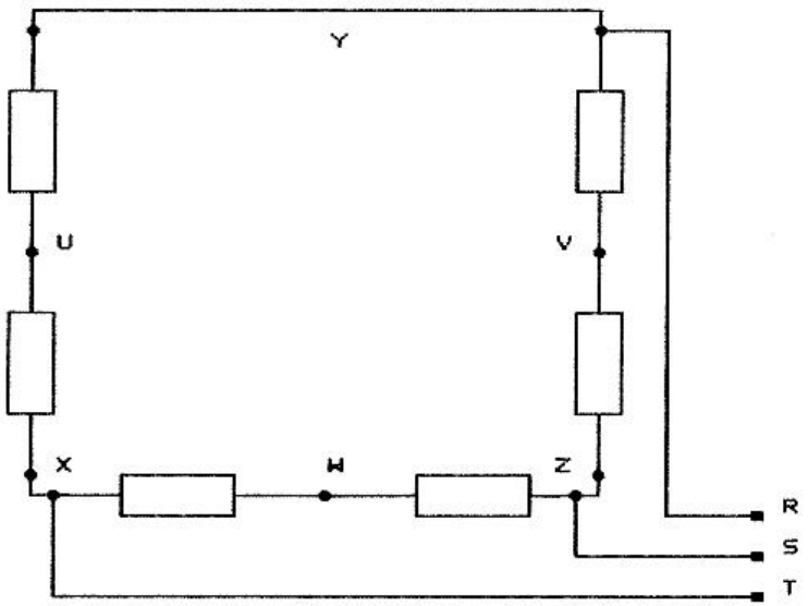
Collegamento D (triangolo) rotazione alla velocità inferiore
