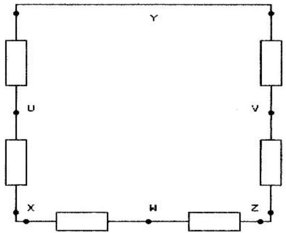
Collegamenti interni tra i semiavvolgimenti
