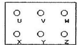
Disposizione collegamenti in morsettiera
